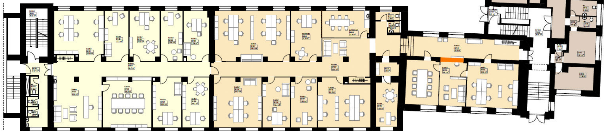
VARIANT C B KORPUS / 1 KORRUS / 1 BÜROO
