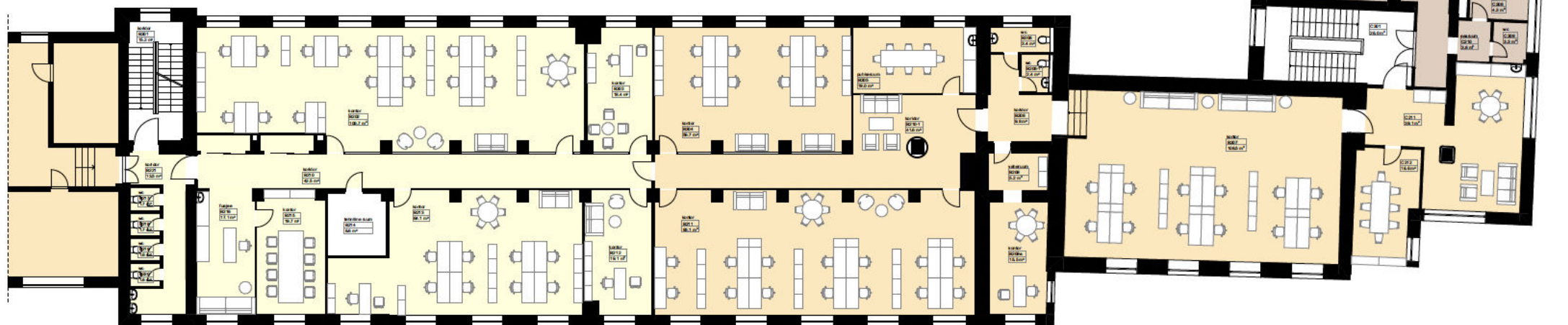
VARIANT C B KORPUS / 2 KORRUS / 2 BÜROO
